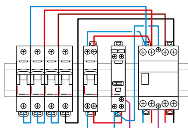
Spínanie trojfázového výkonového stýkača.
