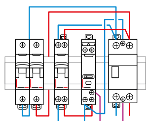
Spínanie jednofázového výkonového stýkača.
