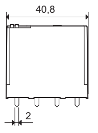
Typ 56.44
