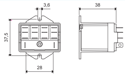
056.45 s relé
