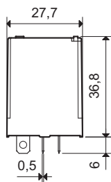
Typ 56.32-0300
