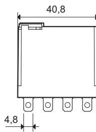
Typ 56.34
