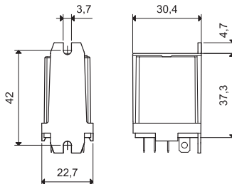
056.26 s relé
